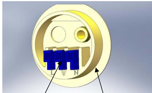
клемник клемная крышка
